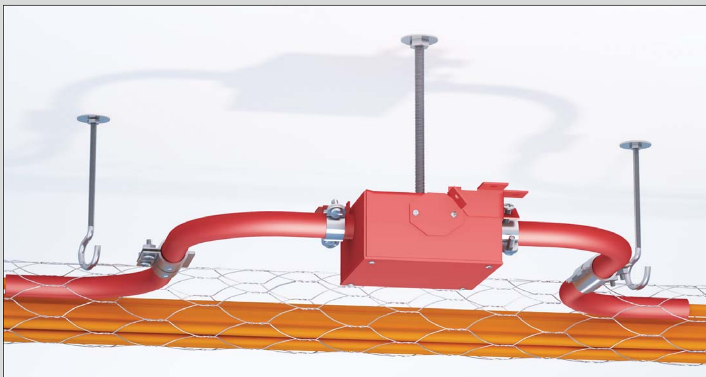
Рис. 21. Пример монтажа ОКЛ «СПЕЦКАБЛАЙН-K2» с монтажной коробкой
