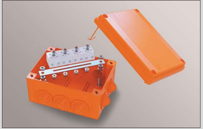
Рис. 25. Огнестойкая монтажная коробка «ДКС»
