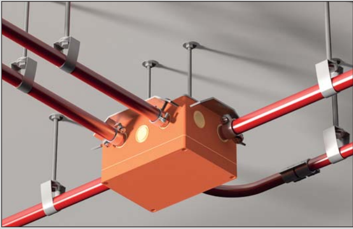
Рис. 24. Пластиковая огнестойкая коробка KSK
