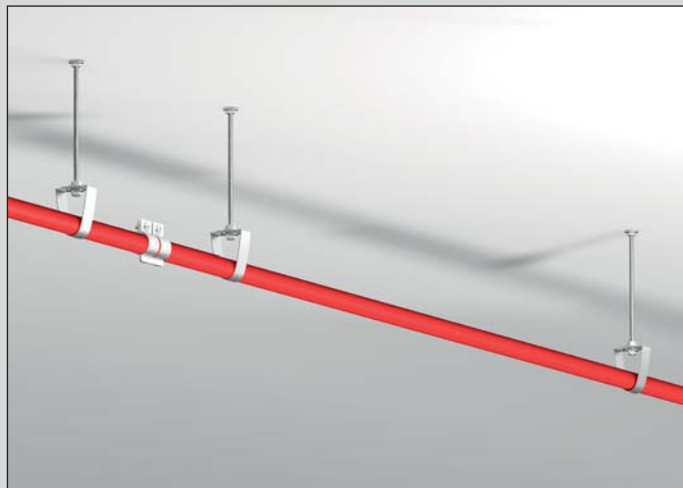
Рис. 17. ОКЛ «СПЕЦКАБЛАЙН-Т», крепление к потолку (одиночная прокладка)
