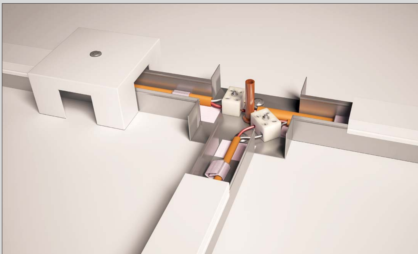
Рис. 18. ОКЛ «СПЕЦКАБЛАЙН-ГЕФЕСТ» (вариант-ККМО)
