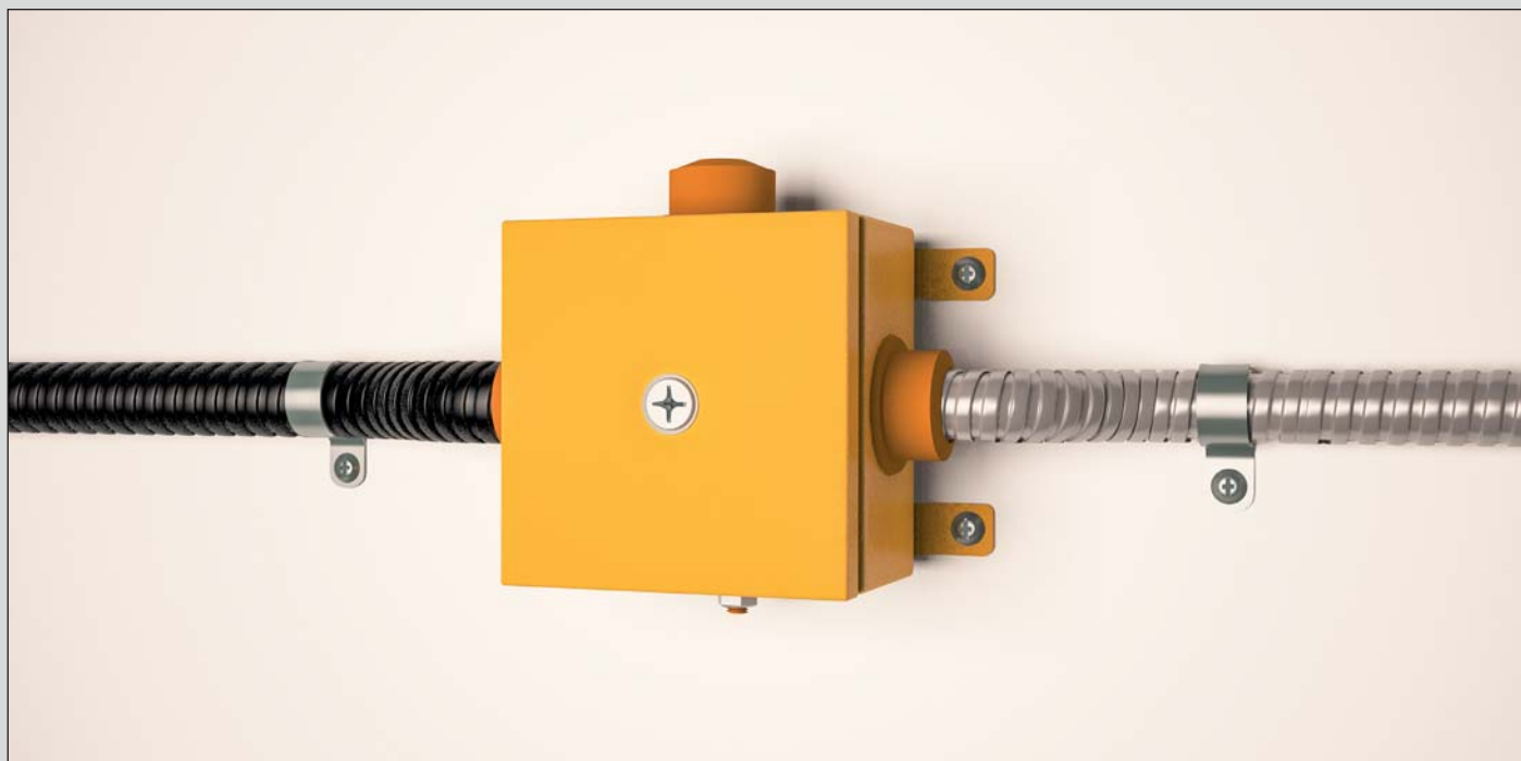
Рис. 7. ОКЛ «СПЕЦКАБЛАЙН-КиТ» в металлическом рукаве
