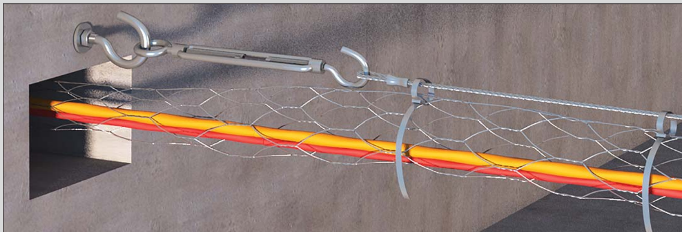
Рис. 11. ОКЛ «СПЕЦКАБЛАЙН-Тр»
